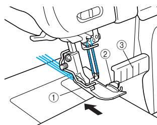
① Pied de biche ② Couteau supérieur ③ Guide de tolérance de couture
