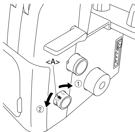
① Inférieur à 1,0 ② Supérieur à 1,0 <Repère de sélection A>
