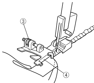
③ Stelschroef ④ Stofgeleider
