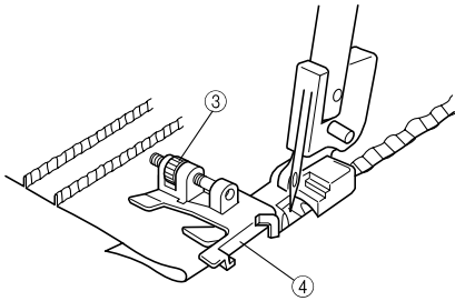
③ Stelschroef ④ Stofgeleider
