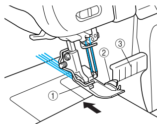
① Persvoet ② Bovenste mesje ③ Geleider voor evenwijdige naden
