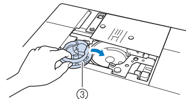
① Marque ▲ sur le boîtier de canette ② Marque ● sur la machine ③ Boîtier de canette
