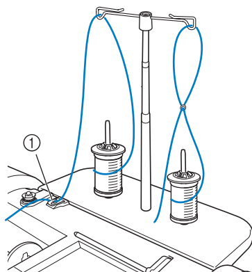
① Guide-fil
