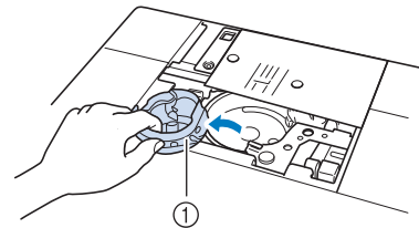
① Boîtier de canette
