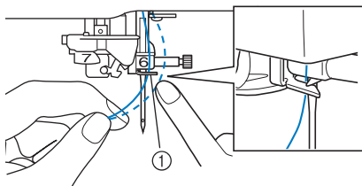
① Guide-fil de la barre de l'aiguille
