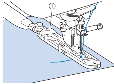
① Plaque du support de bouton
