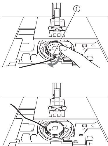
① Ressort de tension
