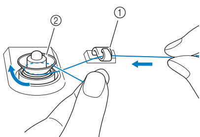
① Guide-fil ② Disque de pré-tension
