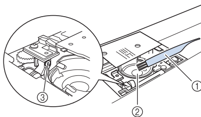
① Brosse de nettoyage ② Coursière ③ Capteur de fil de canette
