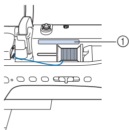
① Voyant lumineux du support pour porte-bobines
