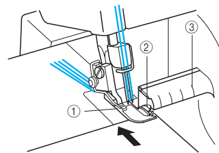
① Persvoet ② Bovenste mesje ③ Geleider voor evenwijdige naden
