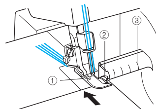
① Pied de biche ② Couteau supérieur ③ Guide de tolérance de couture
