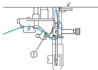
① Rainure du guide-fil
